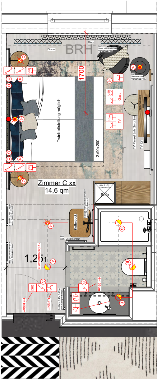
Grundriss Standard Zimmertyp C
