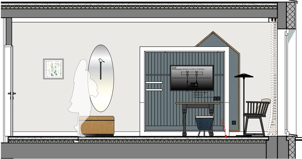
Ansicht TV Paneel Zimmertyp A
