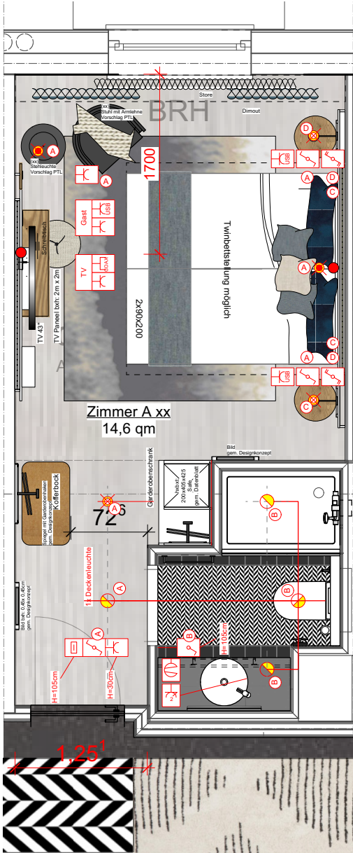
Grundriss Standard Zimmertyp A
